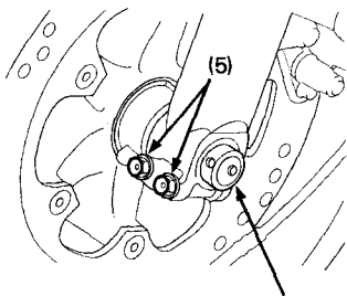
(5) Achsklemmschrauben (6) Vorderachse
