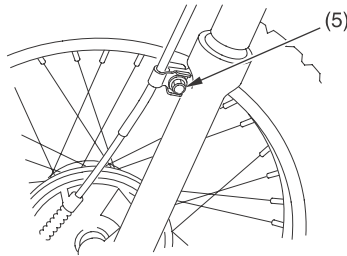
(5) cable guide bolt
