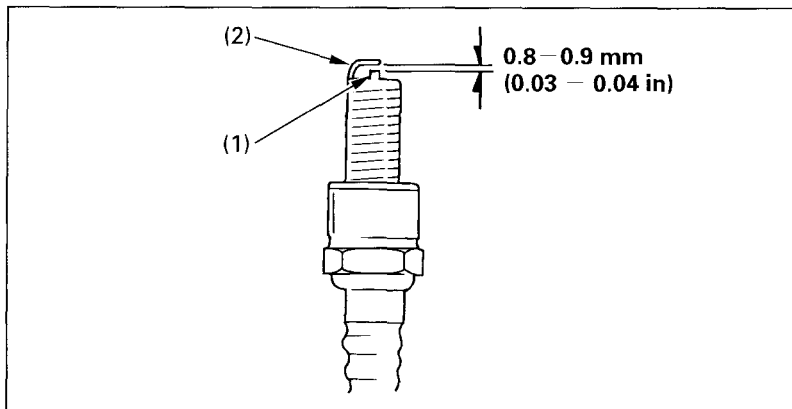
Fig. 4-17 (1) Center electrode
