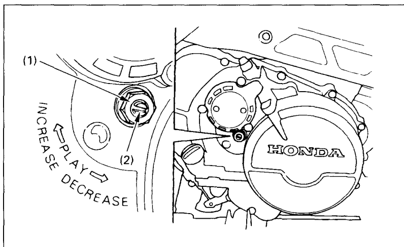
Fig. 4-18 (1) Lock nut
